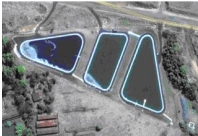
Figura 3. Sistema de Lagoa de estabilização
