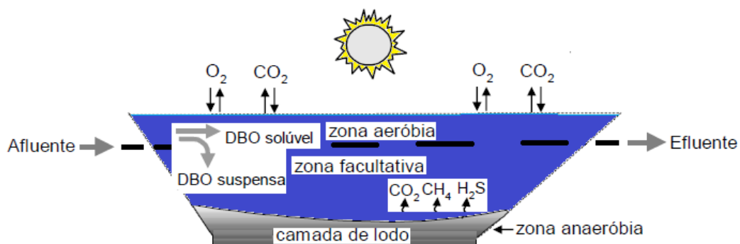
Figura 1. Esquema simplificado de uma lagoa de estabilização
